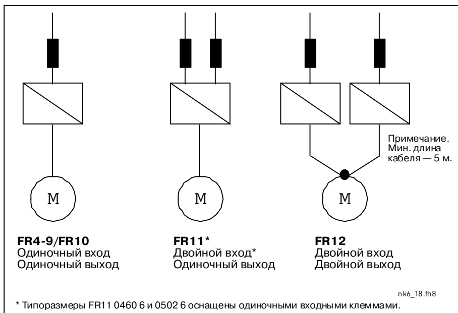
Рисунок 6-1. Топология типоразмеров FR4—FR12
